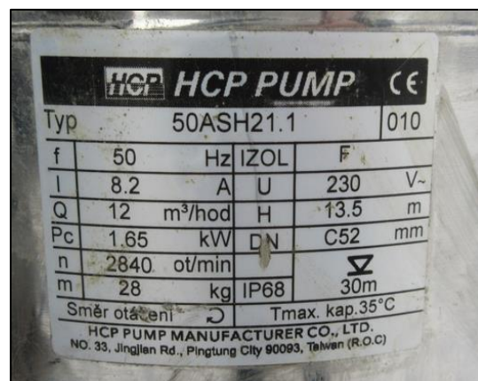
Obrázek 31: Čerpadlo – technický štítek (3. část)
